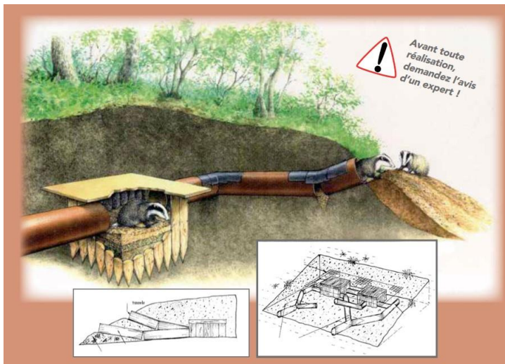
Mise en place des différents éléments du terrier, à l'aval du remblai engraissé - Photo SNCF
